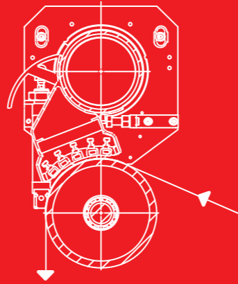
Trajet de la bande pour un dispositif de traitement simple face
